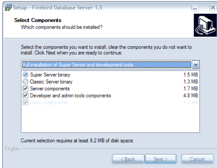
ภาพ 0113 หน้าจอการติดตั้งตามขั้นตอน
